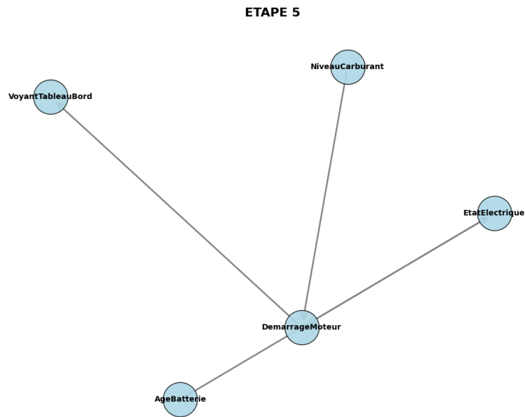
Figure 23: Réseau Bayésien pour le diagnostic de panne de véhicule
